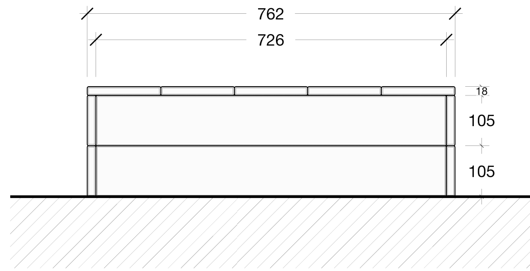
ELEVATION A-A 1:8 @ A3
